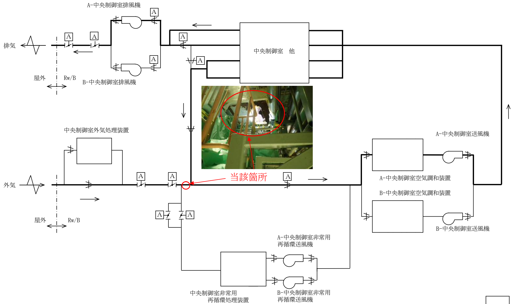
中央制御室空調換気系系統図
