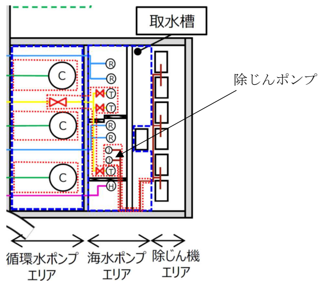
図 2 4 取水槽の除じんポンプの位置（移設前）
