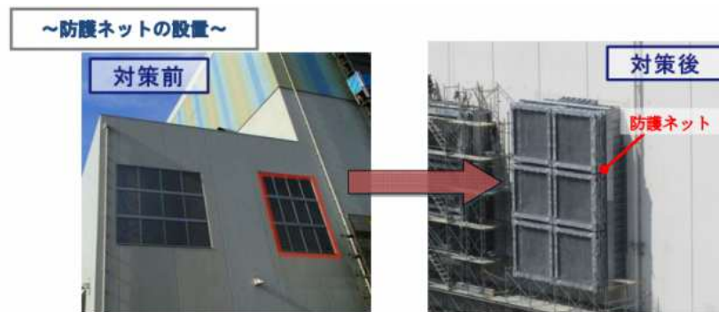
図28 飛来物への対策（竜巻防護ネット）
