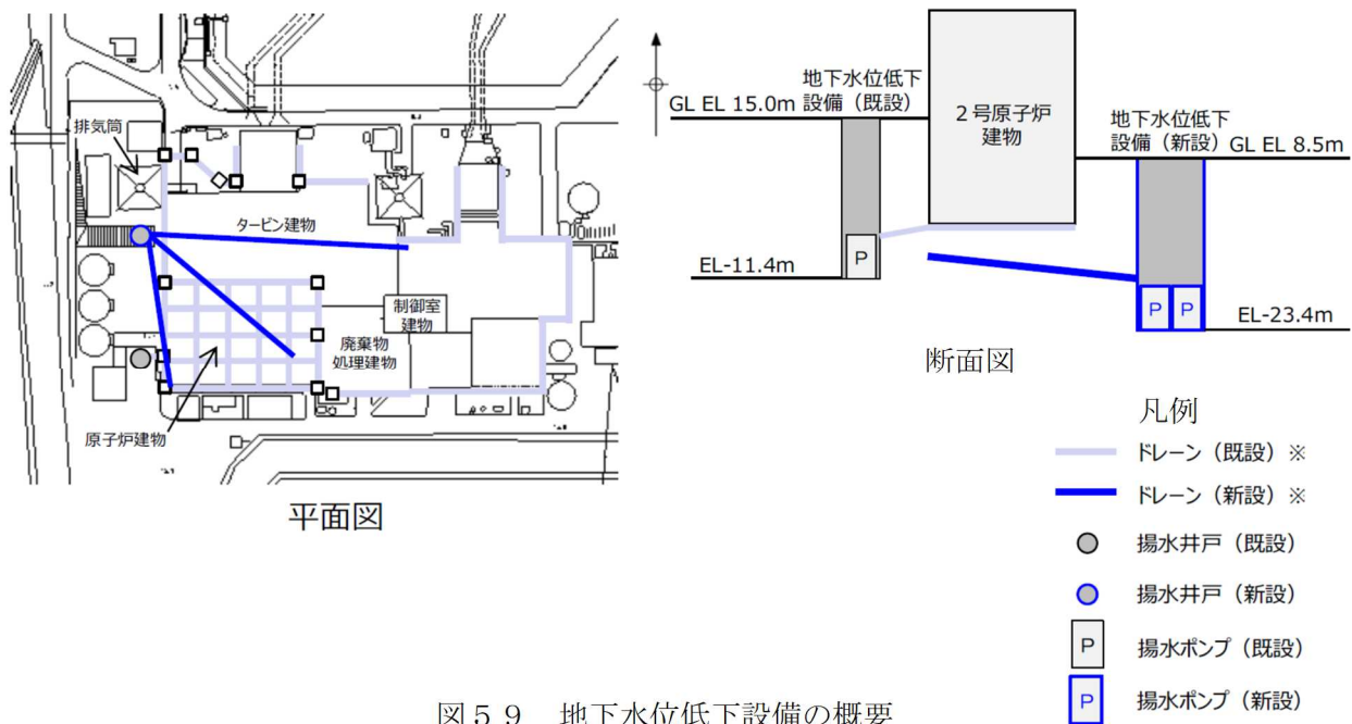
図 5.9 地下水位低下設備の概要
