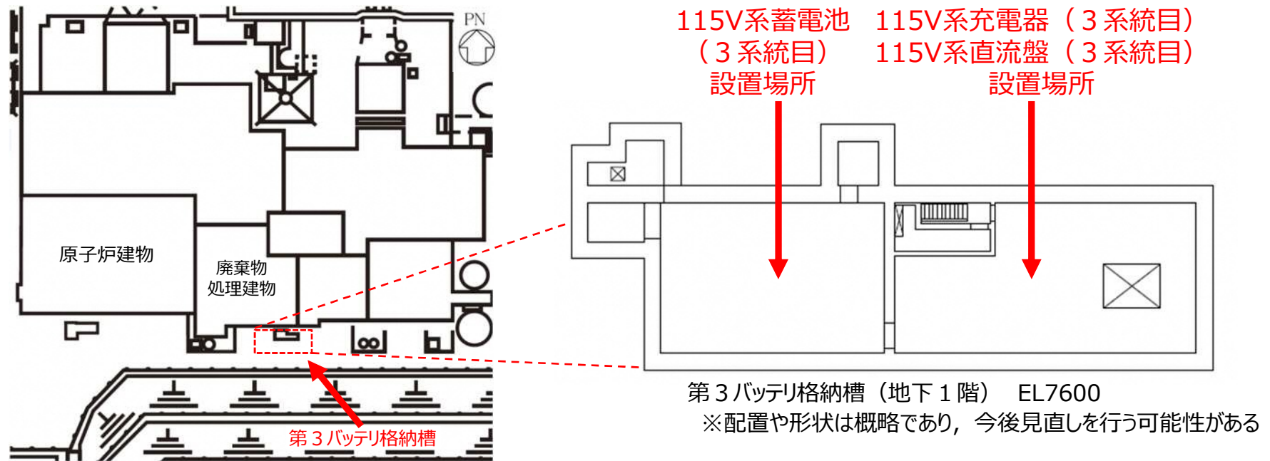
図3 第3バッテリー格納槽配置図
